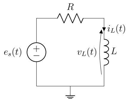
Circuito RL
